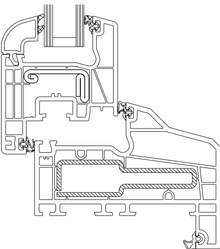
Profieldoorsnede Corona CT 70 Accent met gelijkvallende aanslag (*)
